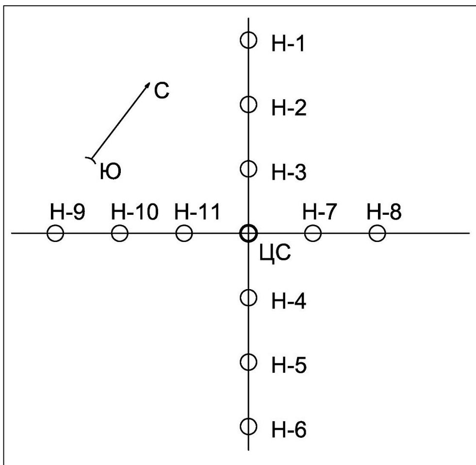
Рис.58. План куста опытной откачки: ЦС – центральная скважина с насосами и фильтрами; H1-H11 – наблюдательные скважины, оборудованные фильтрами
