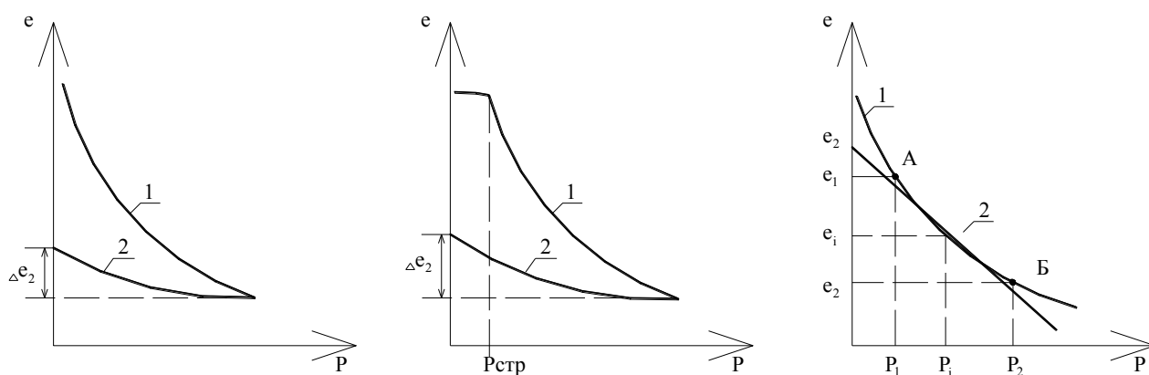
Рис. 66. Компрессионные кривые в координатах «давление – коэффициент пористости»; 1 – кривая уплотнения, 2 – кривая разуплотнения; P_{стр.} – структурная прочность грунта; \Delta e_2 – частичное «восстановление» коэффициента пористости после разгрузки; а) – испытание образца грунта нарушенной структуры; б) – то же, ненарушенной; в) – расчетная схема для участка А–Б компрессионной кривой.
