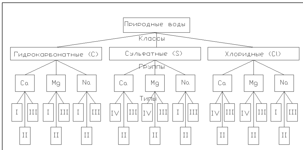
Рис.69. Классификация природных вод по химическому составу (по О.А. Алексиному, 1970)
