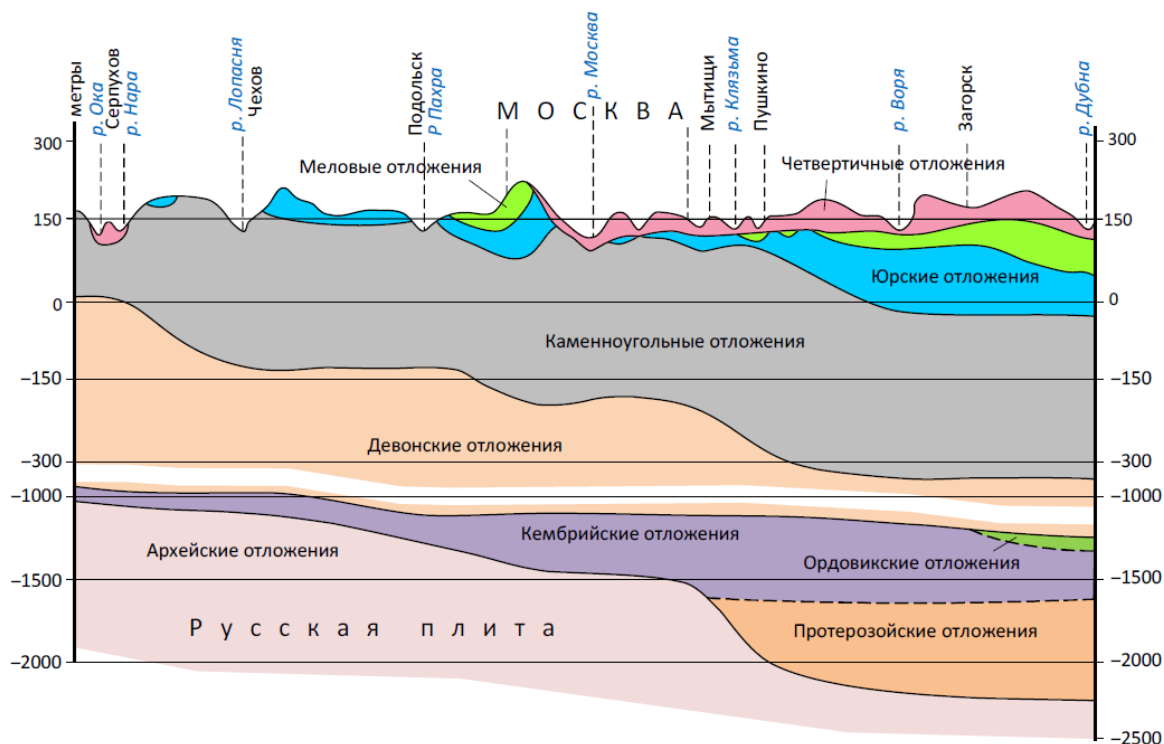
Рис. 5. Схематический геологический разрез по линии р. Ока – Москва – р. Дубна (составили В.М. Соколовский, Е.Н. Мышецкая, 1964)
