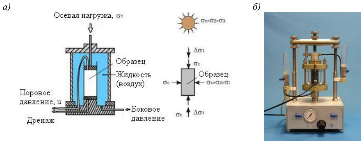
Рис. 67. Стабилметр конструкции ООО «НПП «Геотек», а – конструкция рабочей камеры и схема нагружения образца грунта; б – общий вид прибора
